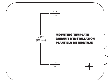
Figure 1 : Servez-vous du gabarit d'installation (inclus).
