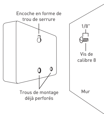
Figure 2 : Accrochez le contrôleur au mur en insérant la vis dans l'encoche en forme de trou de serrure.
