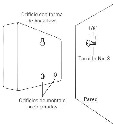
Figura 2: Cuelgue el controlador con un tornillo en el orificio tipo cerradura.
